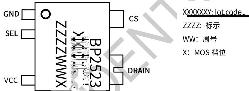
图 2 管脚封装图
